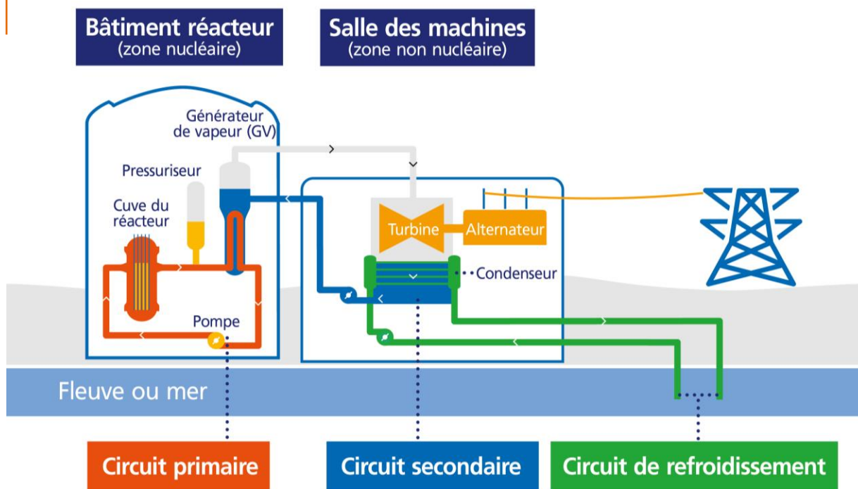
Figure 25. Principes de fonctionnement d'une centrale nucléaire
