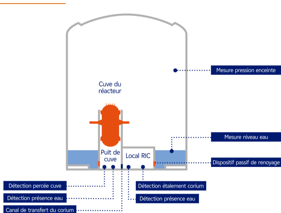
Figure 13. Illustration de la mesure de niveau d'eau dans les puits du bâtiment réacteur et de la détection de l'étalement du corium dans le local d'instrumentation du cœur (RIC)
