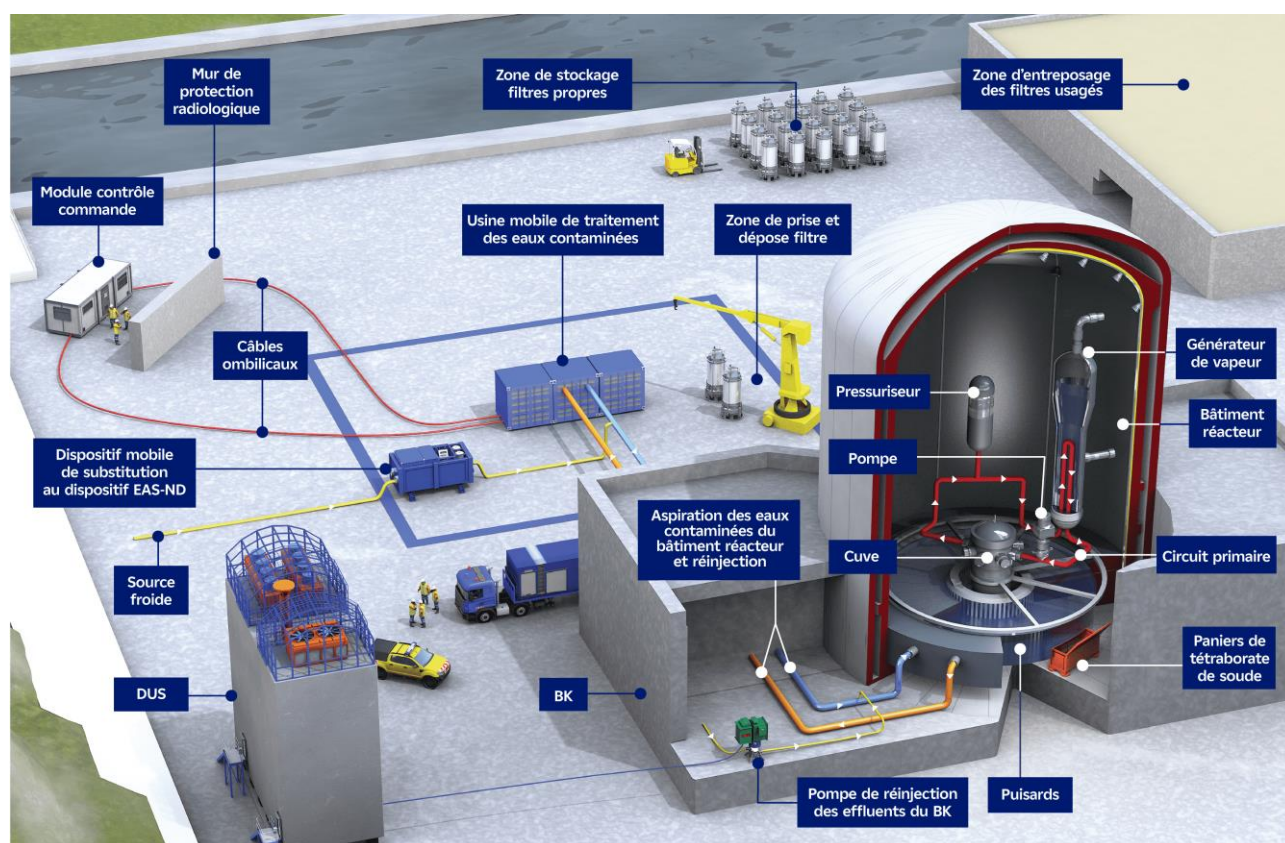
Figure 12. Illustration des dispositions « Lignes fixes pour le traitement des eaux contaminées dans le bâtiment réacteur et modules mobiles de traitement des eaux contaminées », « Mise en œuvre d'une ligne d'injection et d'un dispositif mobile de substitution au dispositif EAS-ND », « Réinjection des effluents du bâtiment combustible dans le bâtiment réacteur », « Mise en place de paniers de tétraborate de diSodium décahydraté dans les puisards du bâtiment réacteur »
