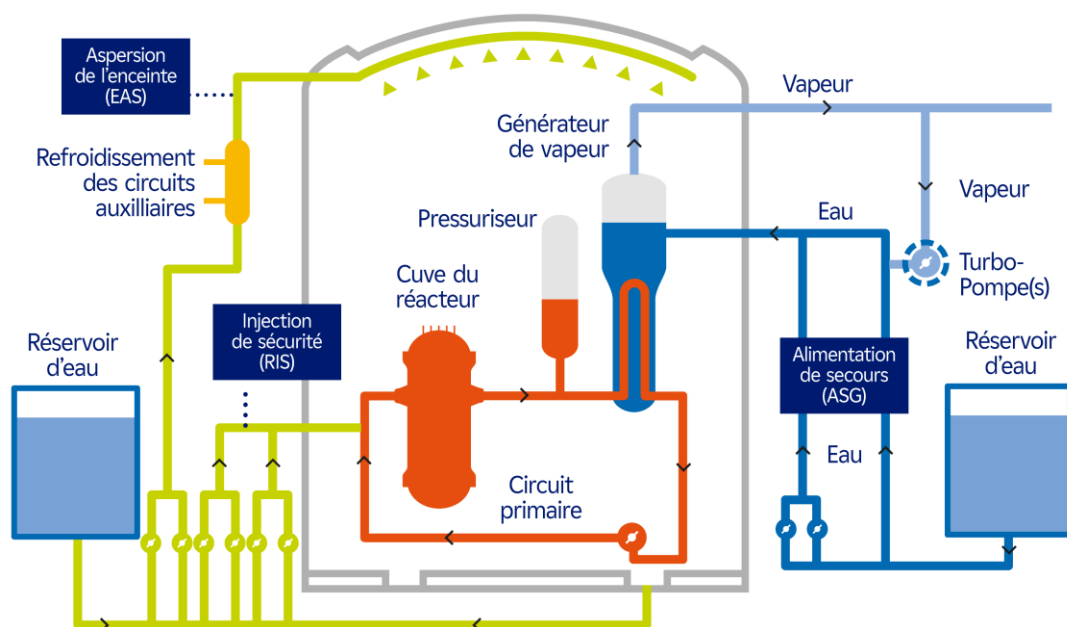
Figure 27. Systèmes de sauvegarde : 3 principaux circuits (ASG, RIS, EAS)
