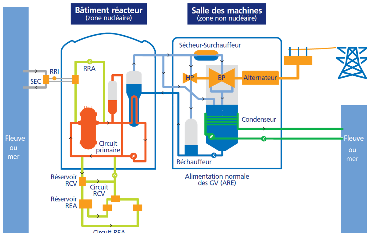
Figure 26. Réacteur en fonctionnement normal : principaux circuits
